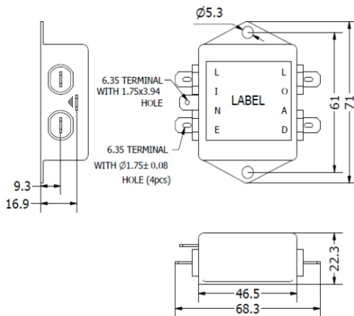
3,4 & 6 Amp Faston Terminal
